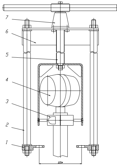
Рис.1 Лубрикатор
