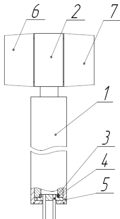
Рис. 1 Модуль измерительный
