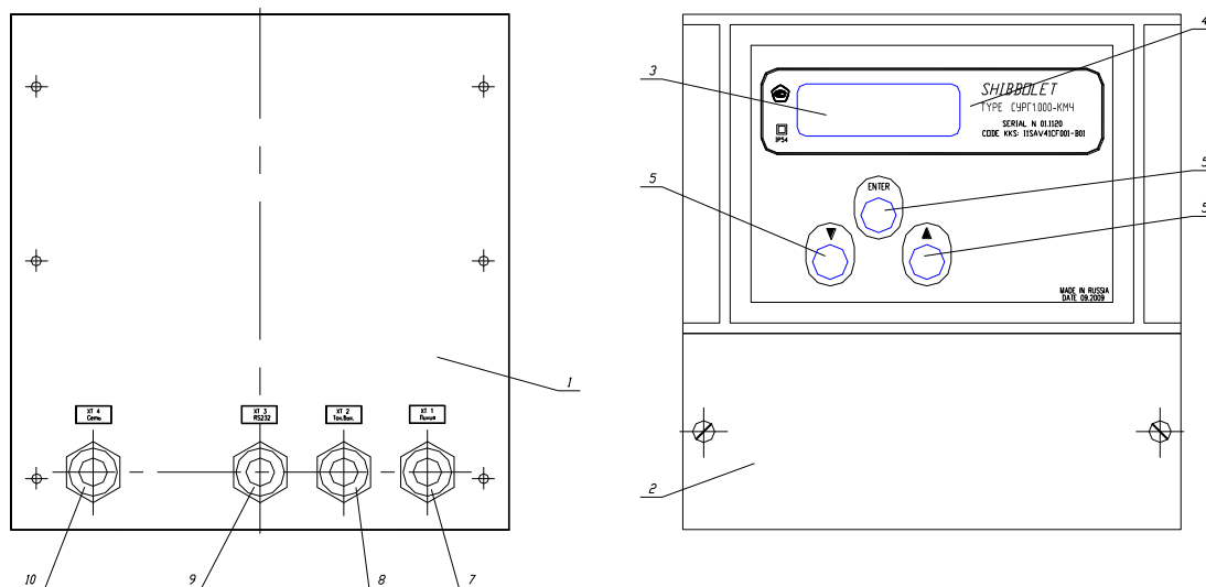
Рис. 2 Внешний вид КВУ
